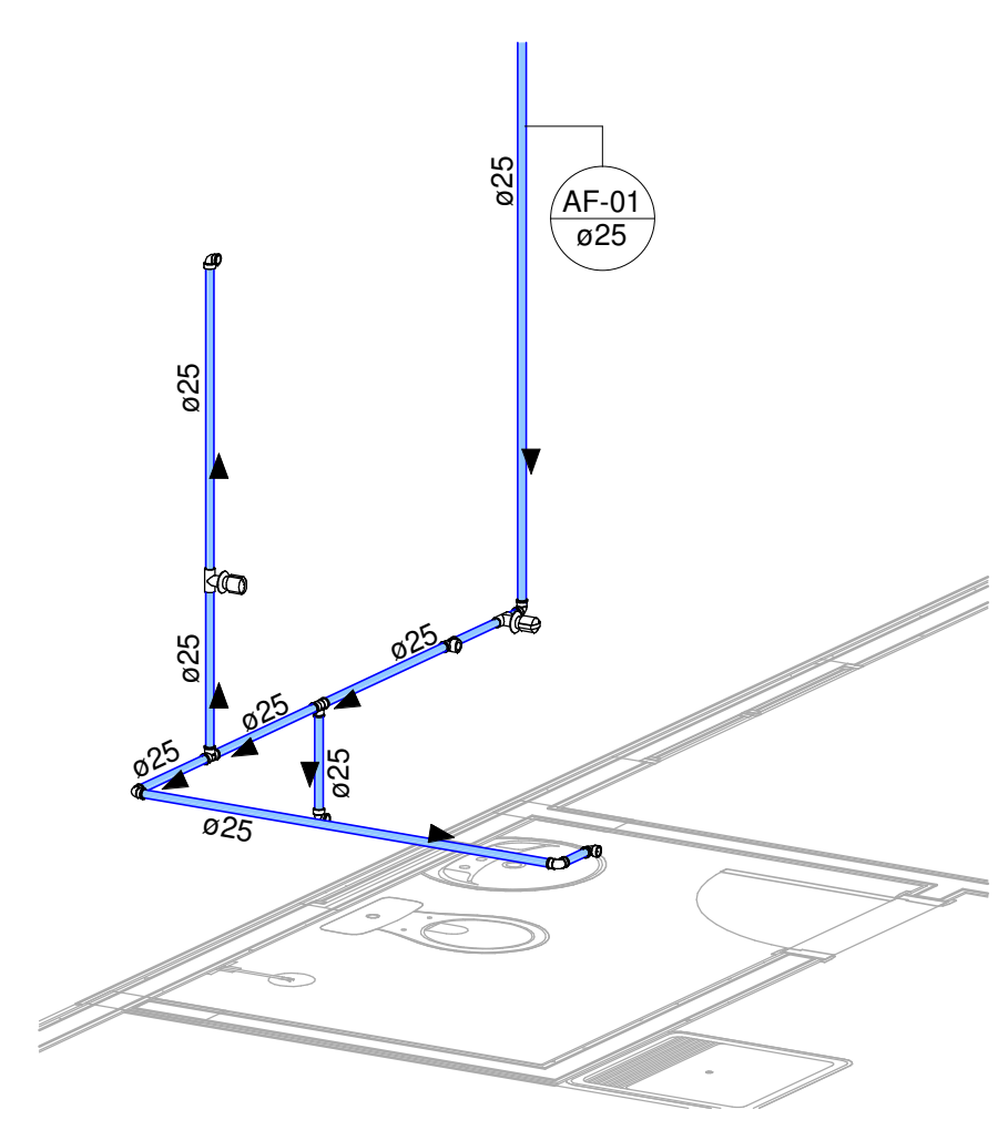
2 Det. 01
